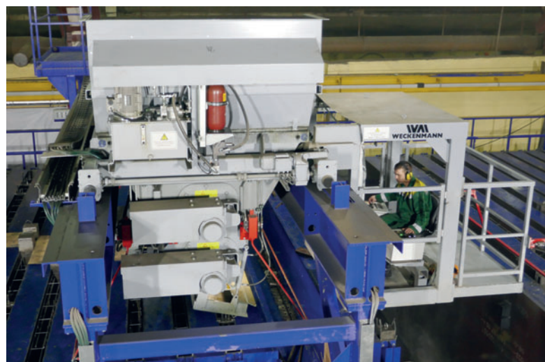
Полупортальный бетонораздатчик при укладке бетона
