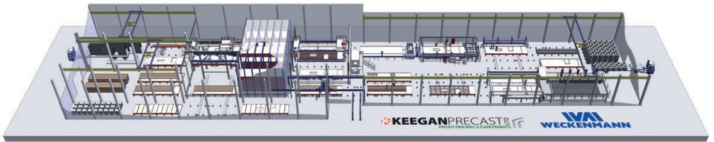
新设备的 3D 设计
